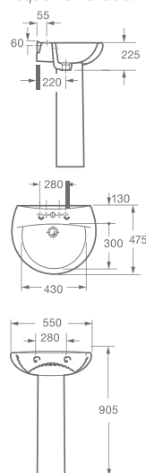
Esquema Lavabo/Pedestal
