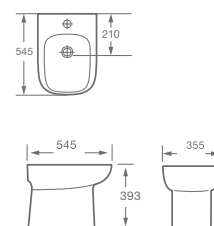
Esquema Bidé
